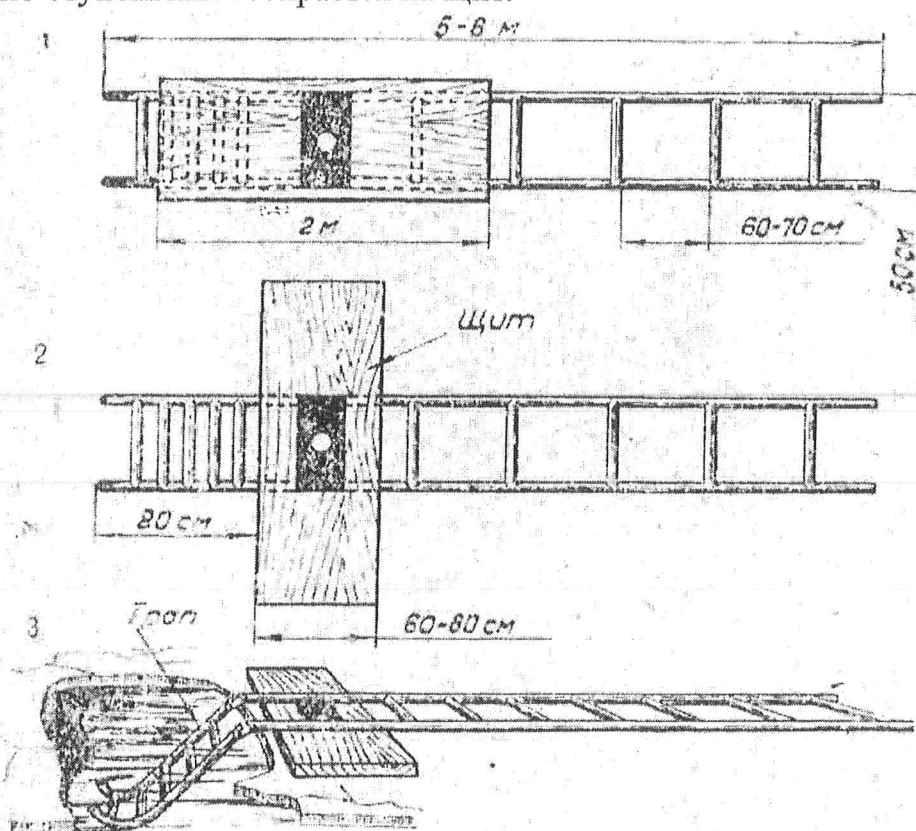
Спасательная лестница № 2
